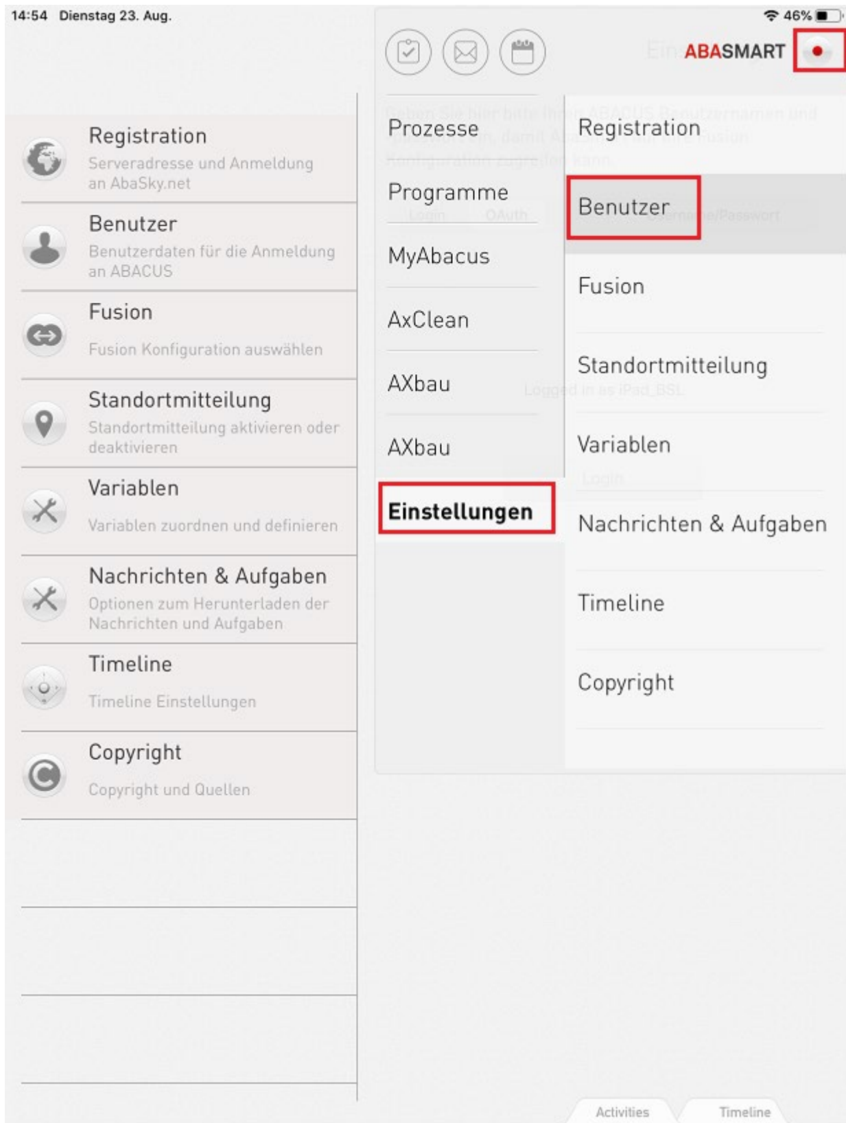
Abbildung 23: Benutzer auf iPad einloggen
